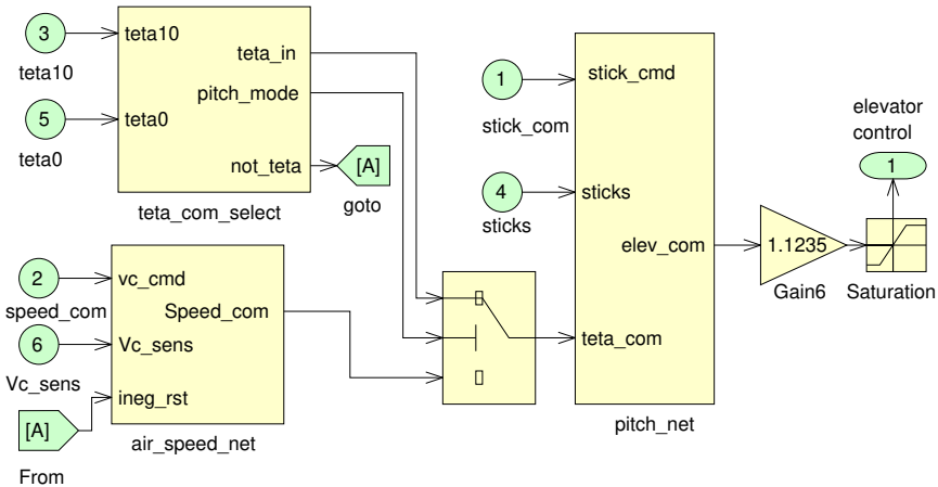
Abb. 2.44 Simulink®-Modell
