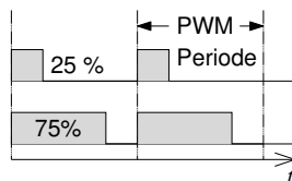
Abb. 3.59 Tastverhältnisse
