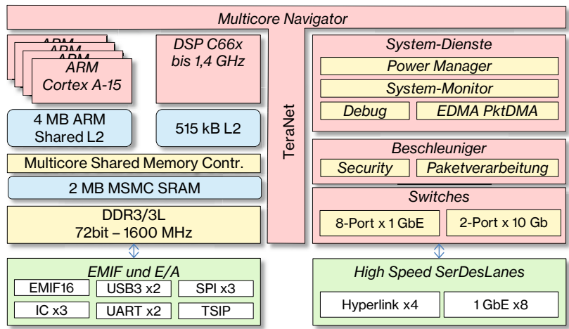
Abb. 3.35 MPSoC 66AK von Texas Instruments® mit ARM®- und C66xxx-Prozessoren ▽
