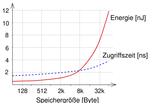
Abb. 3.40 Energieverbrauch und Zugriffszeit für Speicher gemäß CACTI
