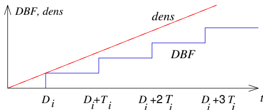
Abb. 6.18 Vergleich von Dichte und DBF
