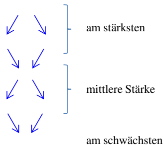
Abb. 2.62 Partielle Ordnung für die Wertemenge {'0', '1', 'Z', 'X', 'H', 'L', 'W'}
