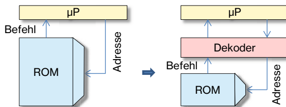
Abb. 3.18 Holen von Befehlen: links : unkomprimiert; rechts : komprimiert
