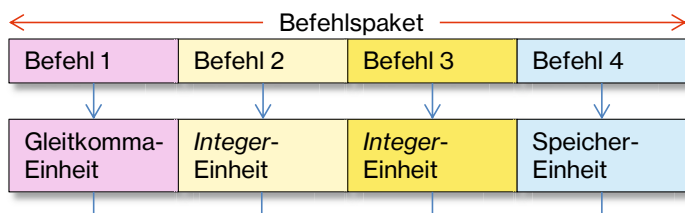
Abb. 3.25 VLIW-Architektur (Beispiel)
