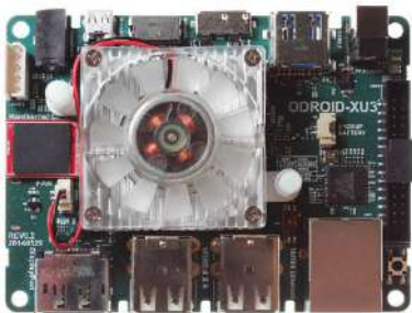
Abb. 5.17 Odroid XU3
