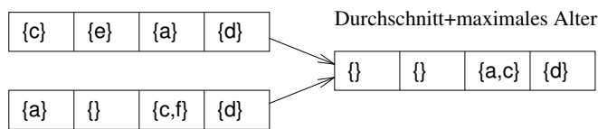
Abb. 5.9 Must-Analyse für LRU-Caches bei rekonvergenten Pfaden
