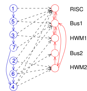
Abb. 6.34 DOL Spezifikationsgraph
