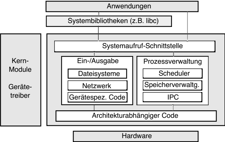
Abb. 4.14 Struktur eines typischen Linux-Systems
