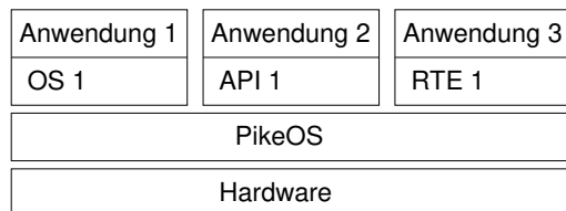
Abb. 4.4 PikeOS-Virtualisierung (©SYSGO)
