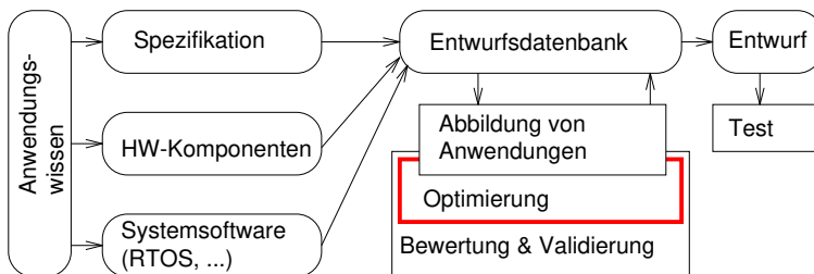
Abb. 7.1 Vereinfachter Entwurfsfluss
