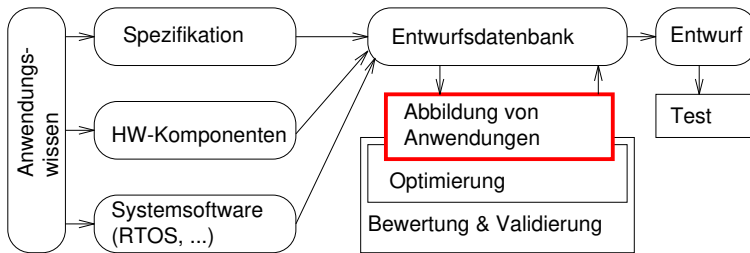
Abb. 6.1 Vereinfachter Entwurfsfluss
