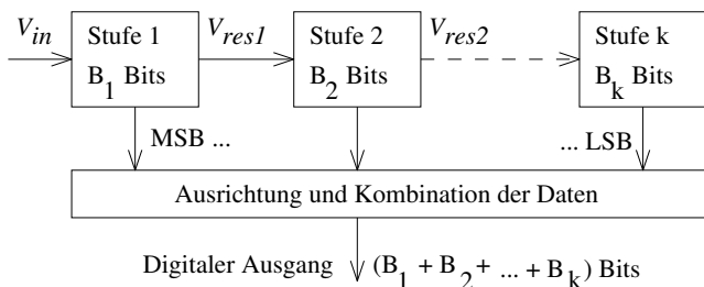
Abb. 3.13 Fließband-A/D-Wandler [292]
