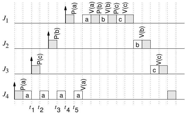
Abb. 4.12 Zweites PCP-Beispiel
