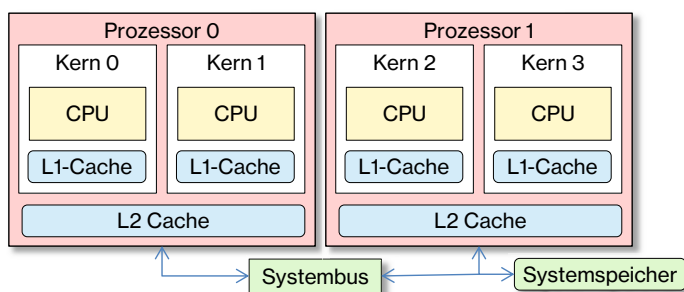
Abb. 3.27 Intel® Core™ Duo-Prozessor
