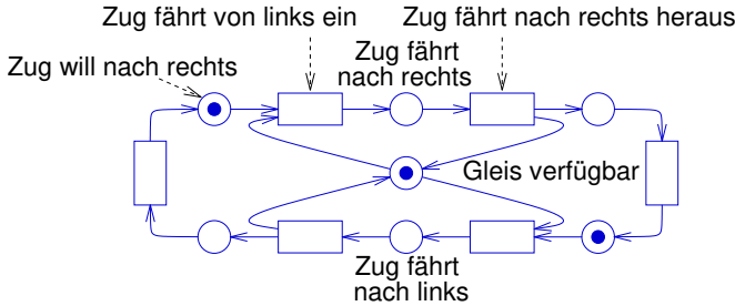
Abb. 2.48 Konflikt um die Ressource „Gleisabschnitt“
