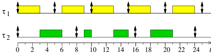
Abb. 6.17 Mit EDF erzeugtes Schedule für das Beispiel aus Abb. 6.14
