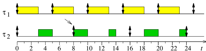
Abb. 6.14 RM-Schedule verpasst die Deadline zum Zeitpunkt 8
