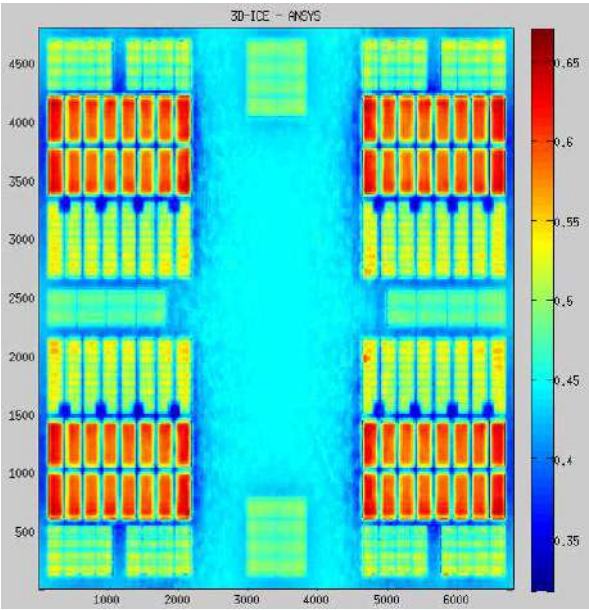
Abb. 5.26 Ergebnisse der thermischen Simulation eines MPSoCs bei 100% Auslastung
