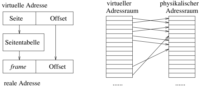
Abb. C.1 Seitenadressierung: links: Adressberechnung; rechts: Abbildung der Adressräume
