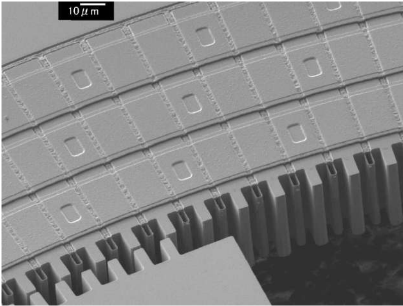
Abb. 3.61 Detail eines rotierenden Schrittmotors; oben: fester Teil, unten: beweglicher Teil; © Sarajlic et al. [478]
