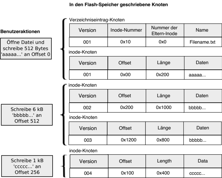
Abb. 4.17 Änderung des Flash-Inhalts bei Schreibvorgängen in JFFS2
