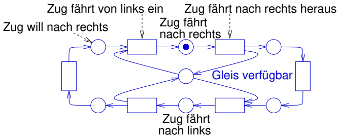
Abb. 2.46 Verwendung der Ressource „Gleisabschnitt“
