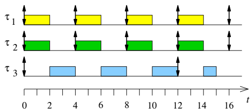
Abb. 6.25 Mit G-RM erzeugtes Schedule verpasst Deadline bei t = 12
