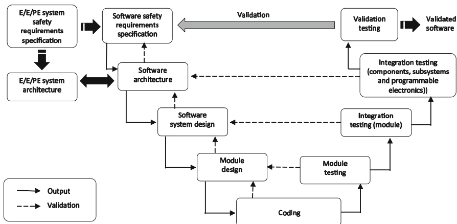
Fig. 1. The V-model
