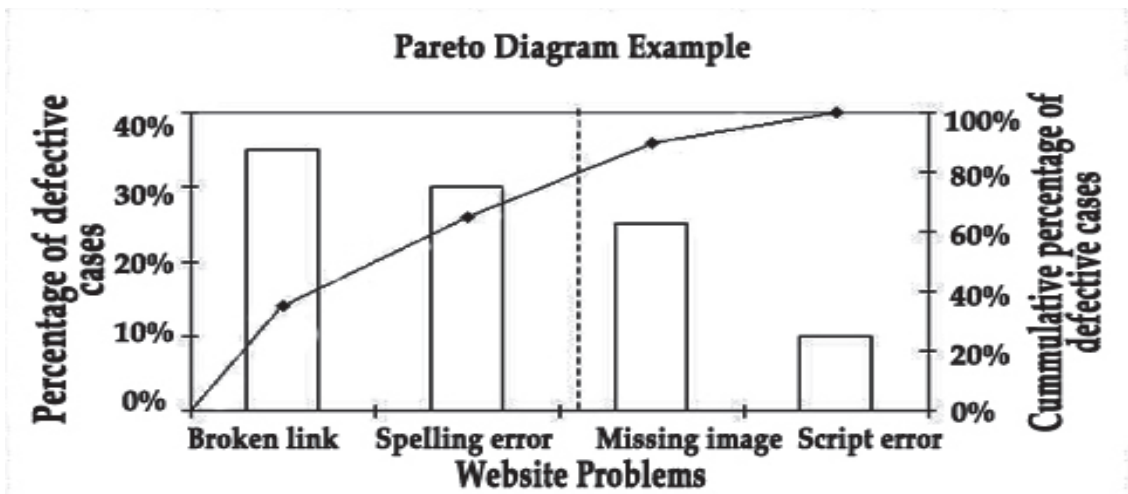
Fig. 9. Pareto diagram
