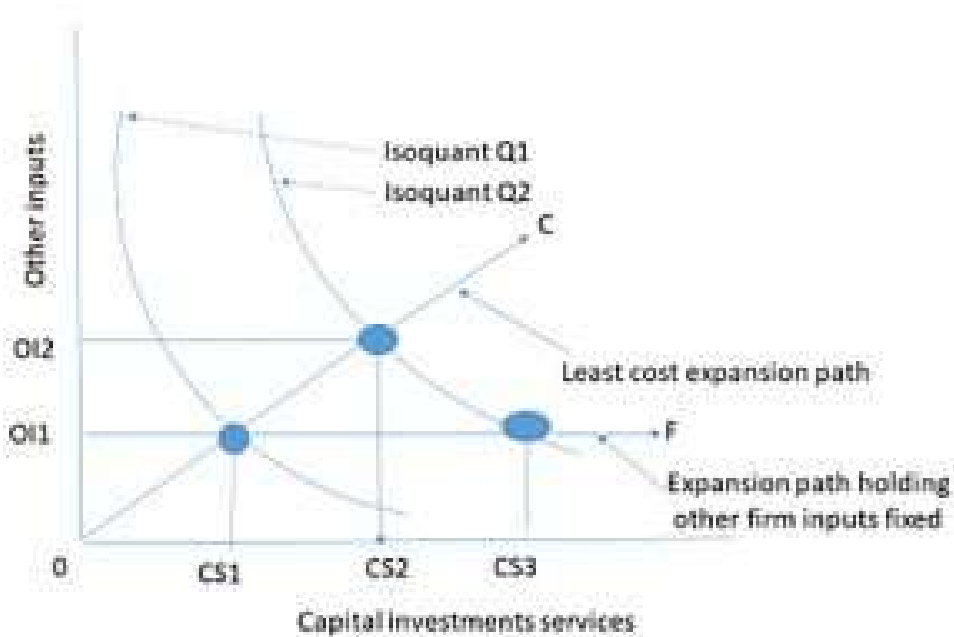
Figure 10.1. Isoquants
