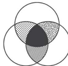
Figure 22.3. Venn diagram.
