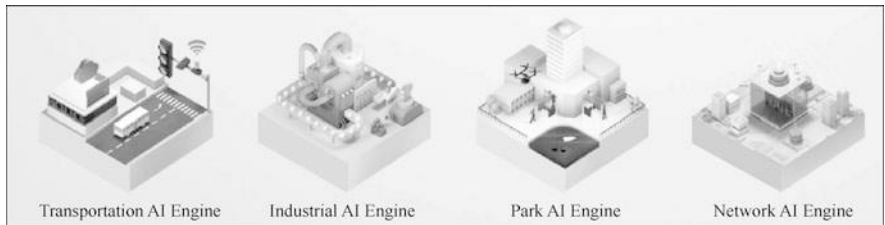
Fig. 8.2 EI agent
