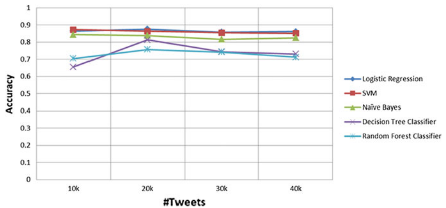
Fig. 10 AUC comparison
