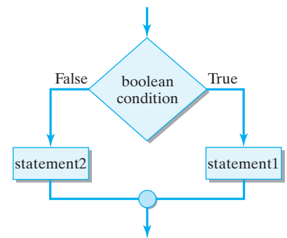
If-else syntax
